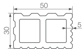
wymiary legara (mm)
