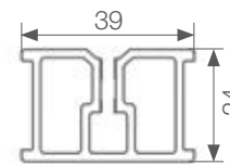
wymiary legara alumiowego (mm)
