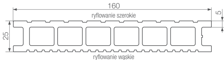
wymiary deski (mm)
