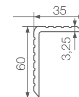
wymiary kompozytowej listwy wykończeniowej (mm)
