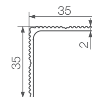
wymiary aluminiowej listwy wykończeniowej (mm)
