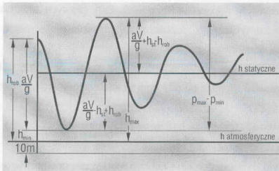
Przebieg fali uderzenia hydraulicznego
