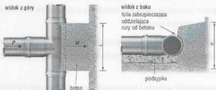
Blok опорowy для трóјника
