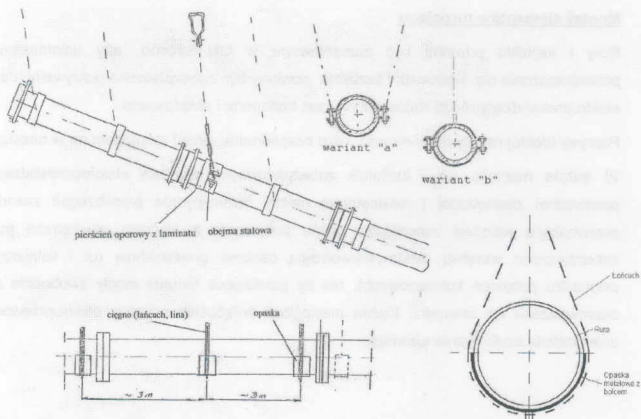
Przykłady mocowania rur na zawiesiach.
