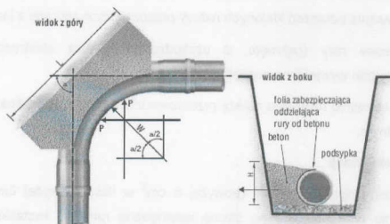
Blok oporowy kolana lub łuku
