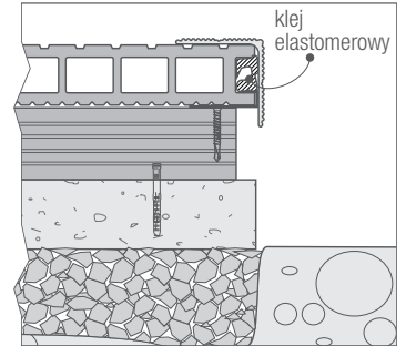
montaż listwy za pomocą kleju elastomerowego
