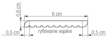
kompozytowa listwa wykończeniowa
