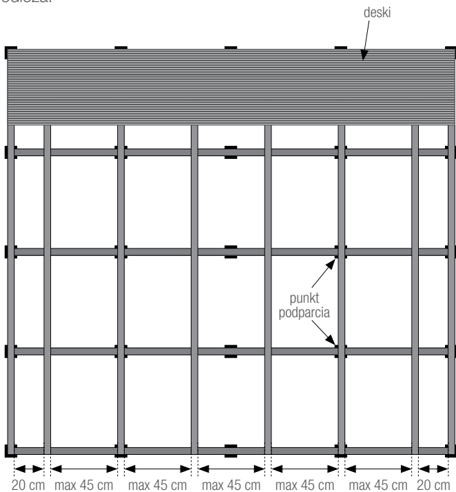
taras pływający na kratownicy metalowej
