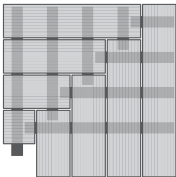
przykładowy układ legarów przy deskach ułożonych w „jodełkę”
