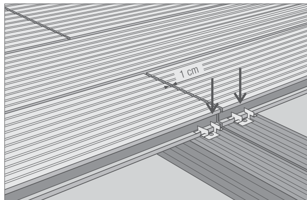
połączenie czołowe desek na dwóch oddzielnych legarach (dylatacja 1 cm)
