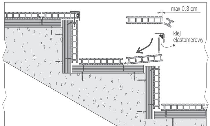
mocowanie desek poziomych prycinanie i montaż z listwą kątową
