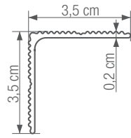
narożna, aluminiowa listwa wykończeniowa
