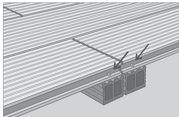
montaż ostatnich desek na wkrętach przykręconych pod kątem
