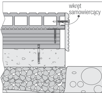
montaż listwy za pomocą wkrętów samowiercących
