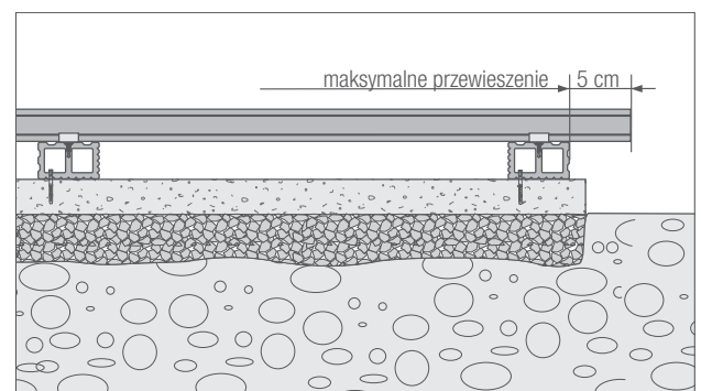
maksymalne wysunięcie deski poza legar 5 cm
