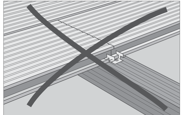
nieprawidłowe łączenie czołowe 2 desek
