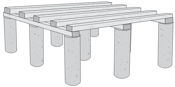
podłoże na gruncie - taras na podporach betonowych z kostką drewnianą
