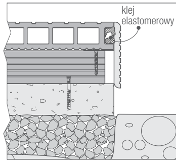
montaż listwy za pomocą kleju elastamerowego
