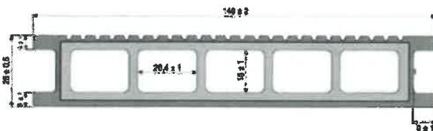
Rys. 2. Deska tarasowa WPC GAMRAT 140x25 jednostronnie ryflowana
