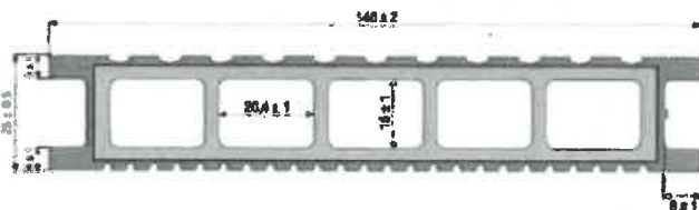
Rys. 3. Deska tarasowa WPC GAMRAT 140x25 dwustronnie ryflowana
