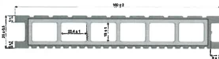
Rys. 1. Deska tarasowa WPC GAMRAT 160x25 dwustronnie ryflowana
