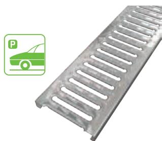
Kratka ze stali ocynkowanej z żebrami poprzecznymi i systemem antypoślizgowym, certyfikowana dla klasy obciążenia B125
