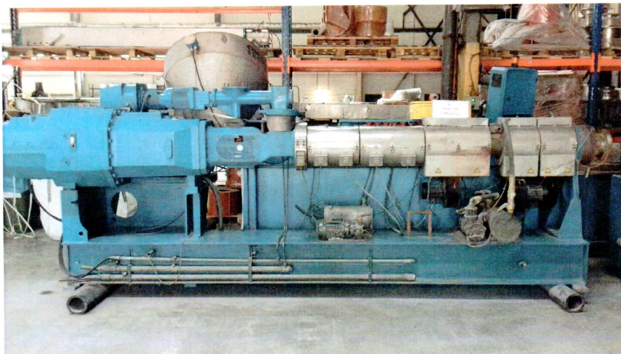
Fot.1 Wytłaczarka dwuślimakowa
