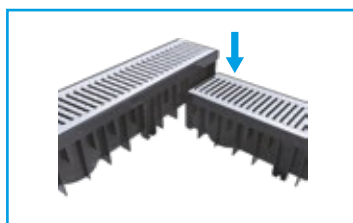
ŁĄCZENIE BOCZNE
