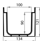
ODWODNIENIE 130/90
